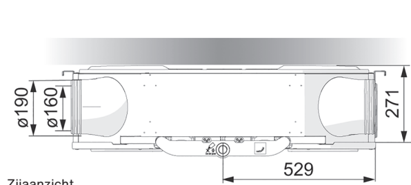
Zijaanzicht
