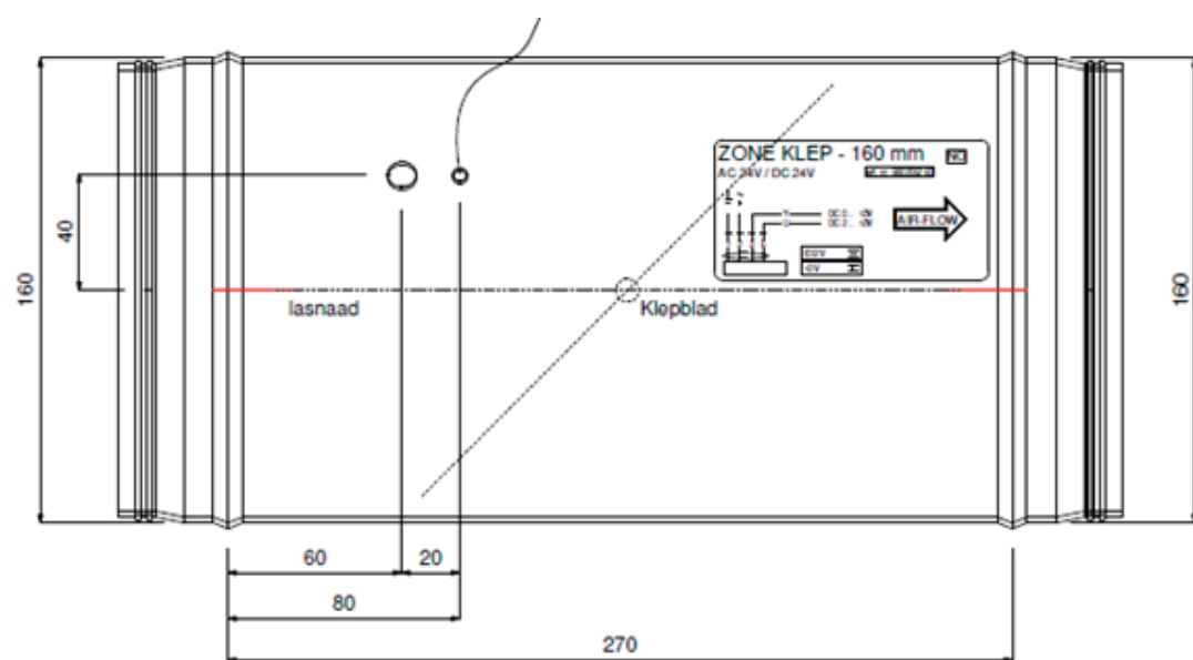
Afbeelding 4.2: Zoneklep Ø160mm
