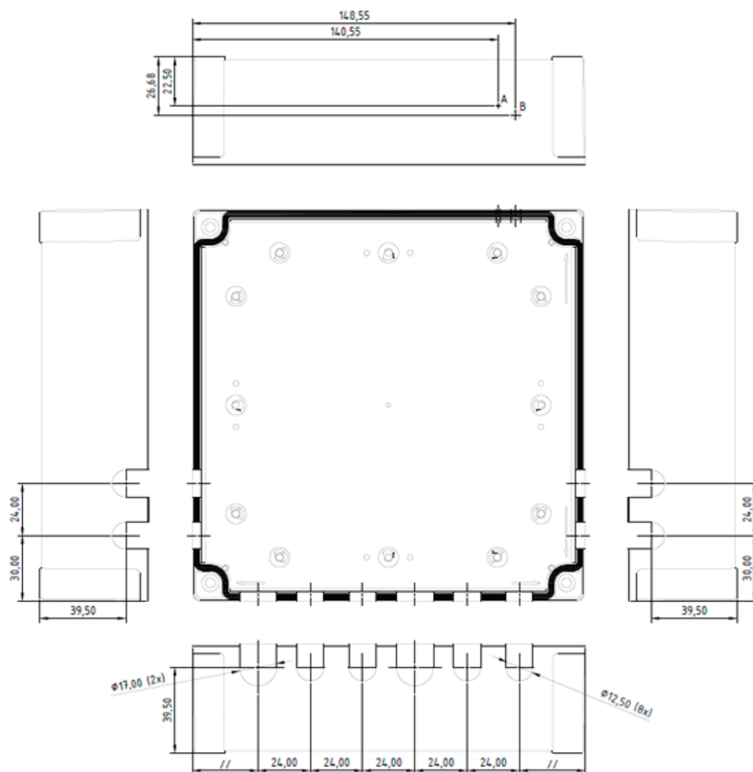
Abbeelding 4.3: ComfoZone Box
