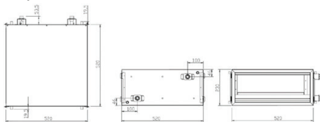
Maatvoering CW 10
