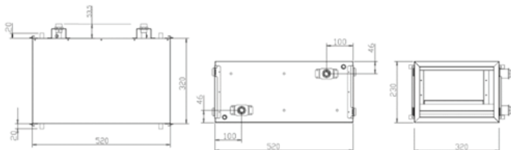
Maatvoering CW 6
