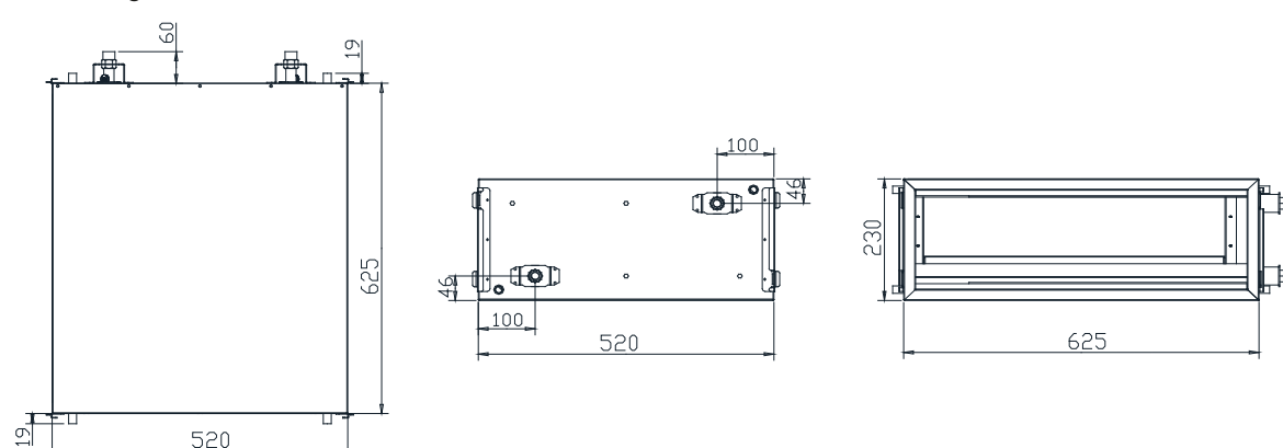
Maatvoering CW 12
