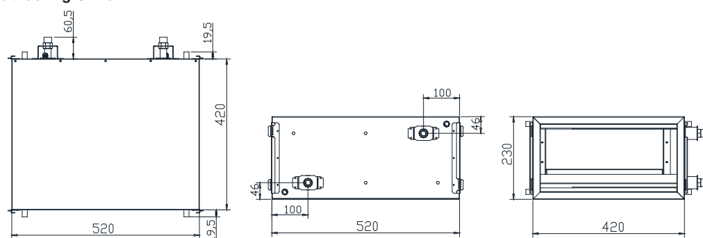
Maatvoering CW 8
