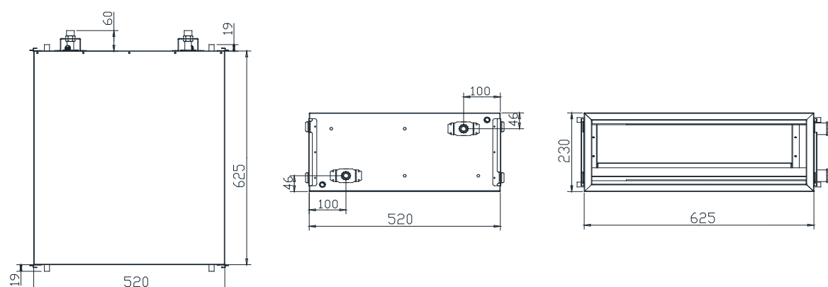
Maatvoering CW 12
