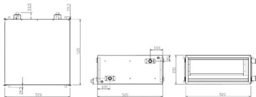
Maatvoering CW 10
