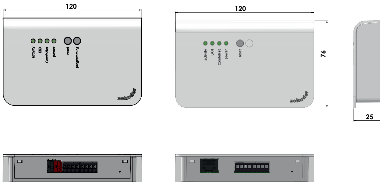
Afbeelding 3.0: Maatschets ComfoConnect
