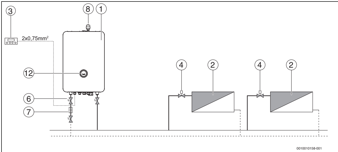
Afb. 37 Alleen cv-bedrijf
