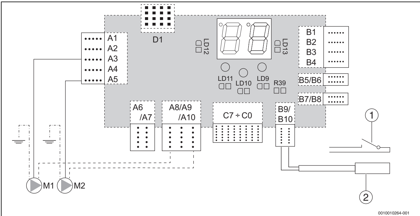
Afb. 28 Sturing van de opwarming van het warmwater door twee pompen (met keerklep)
