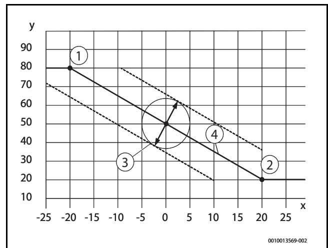
Afb. 33 Weersafhankelijk geregelde stooklijn
