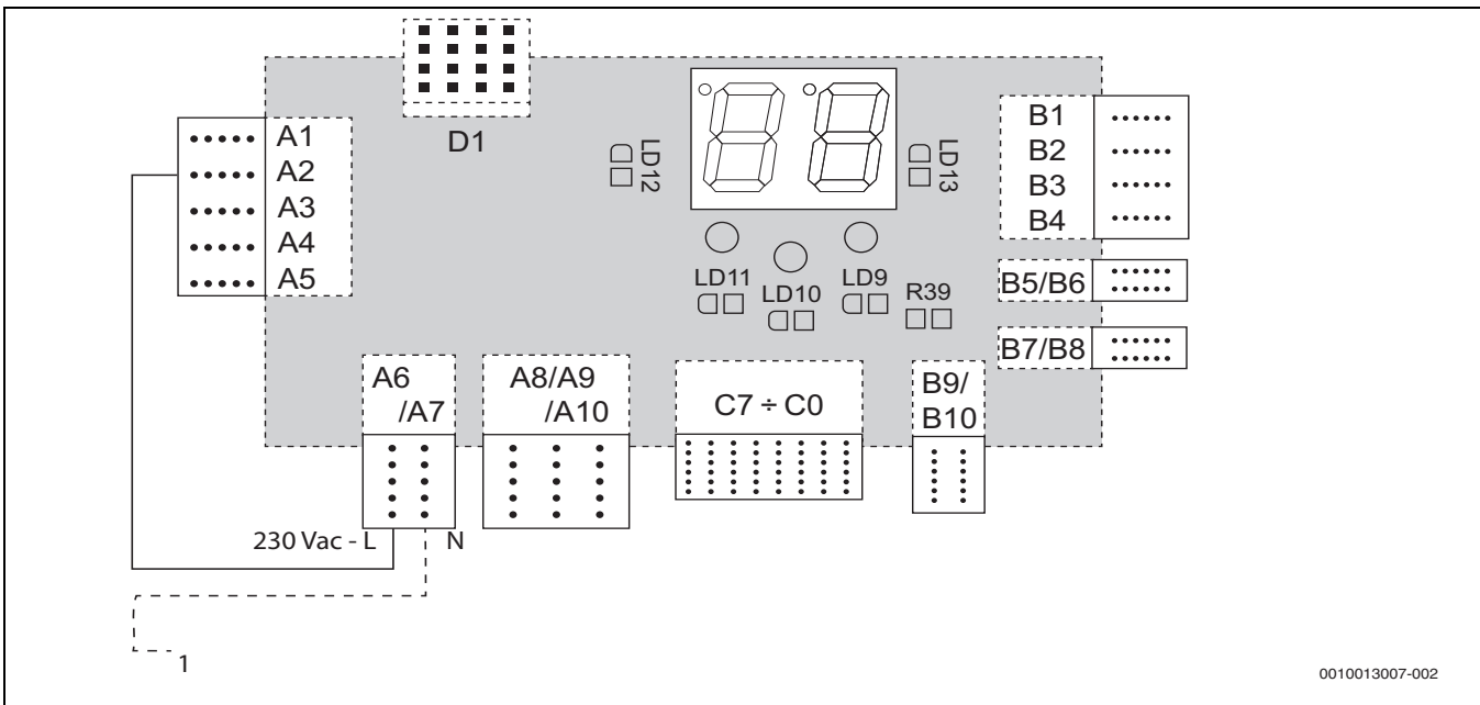
Afb. 24 Sturing van het cv-toestel door regeling warmtedistributie (aparte externe nulgeleider, spanningsvrij geschakeld contact)
