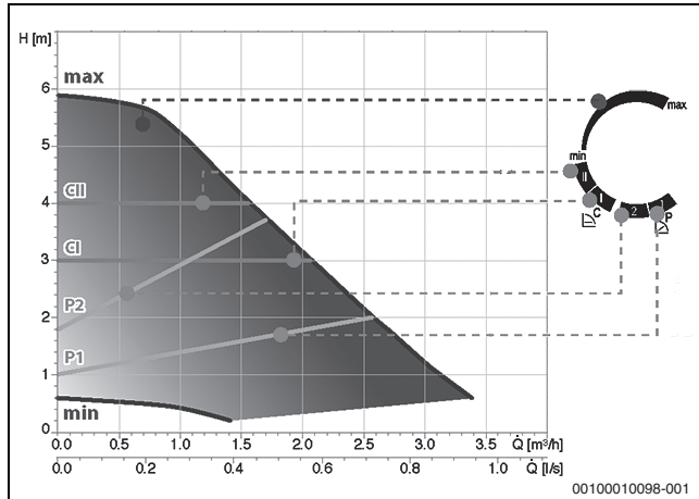
Afb. 34 Opvoerhoogte cv-pomp voor cv-toestel Tronic Heat 3500 4...24 kW
