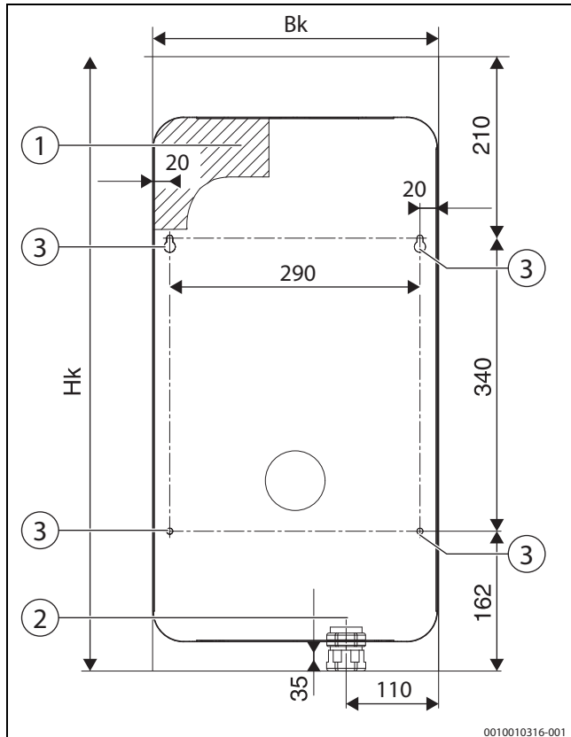
Afb. 8 Afmetingen van de boringen voor de bevestiging van het cv-toestel aan de muur en voor de voedingskabel voor het cv-toestel Tronic Heat 3500 4-12 kW
