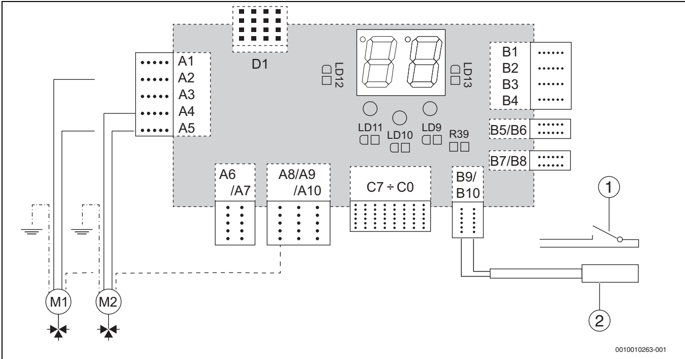
Afb. 27 Sturing van de opwarming van het warmwater via de warmwatertemperatuursensor of het contact van de warmwaterthermostaat
