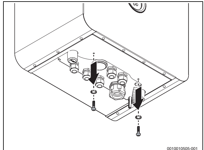
Afb. 6 Draai de schroeven los
