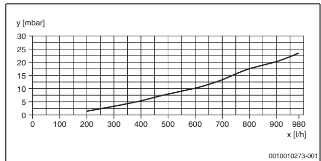
Afb. 36 Hydraulische weerstand Tronic Heat 3500 15...24 kW
