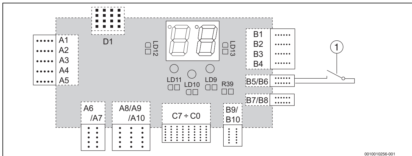
Afb. 20 Aansluiting kamerthermostaat
