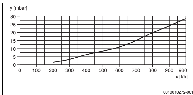
Afb. 35 Hydraulische weerstand Tronic Heat 3500 4...12 kW
