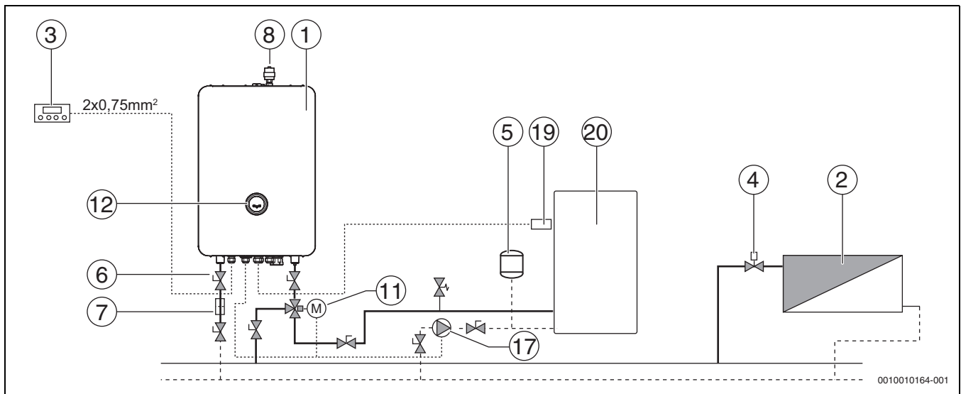
Afb. 39 Voorbeeld van aansluiting van het elektrische cv-toestel Tronic Heat 3500 als vervangende warmtebron
