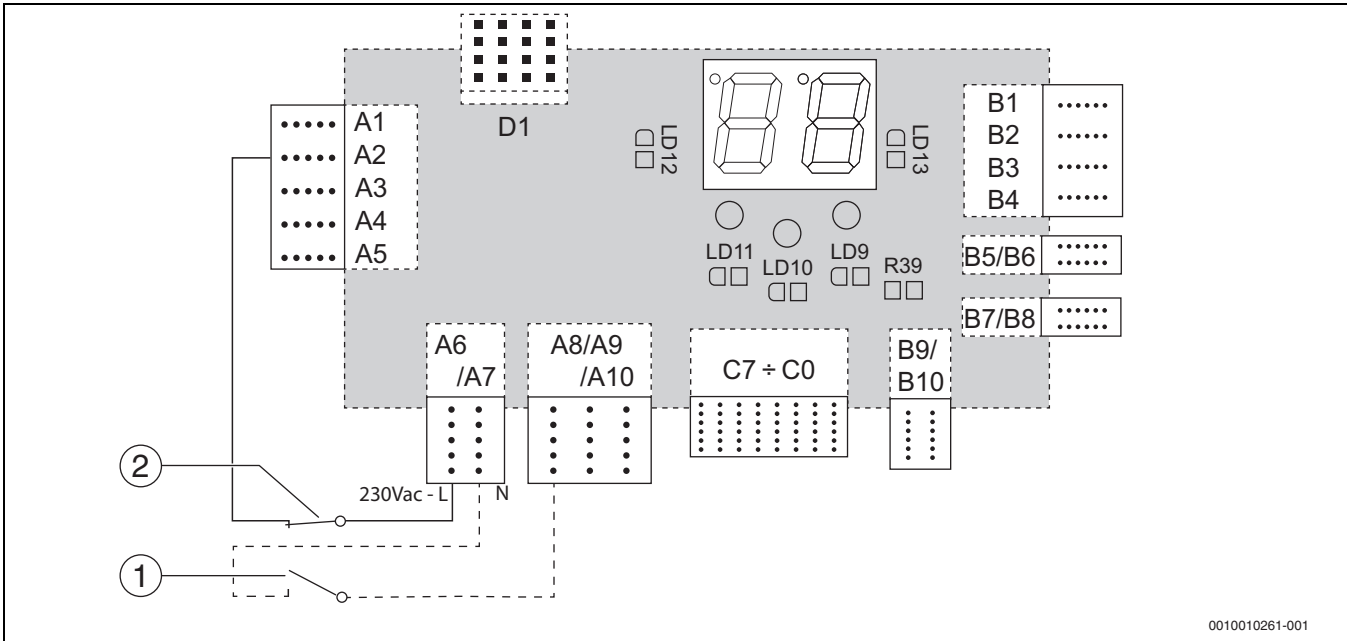
Afb. 23 Blokkeren van het cv-toestel en sturing door regeling warmtedistributie (nulleider)
