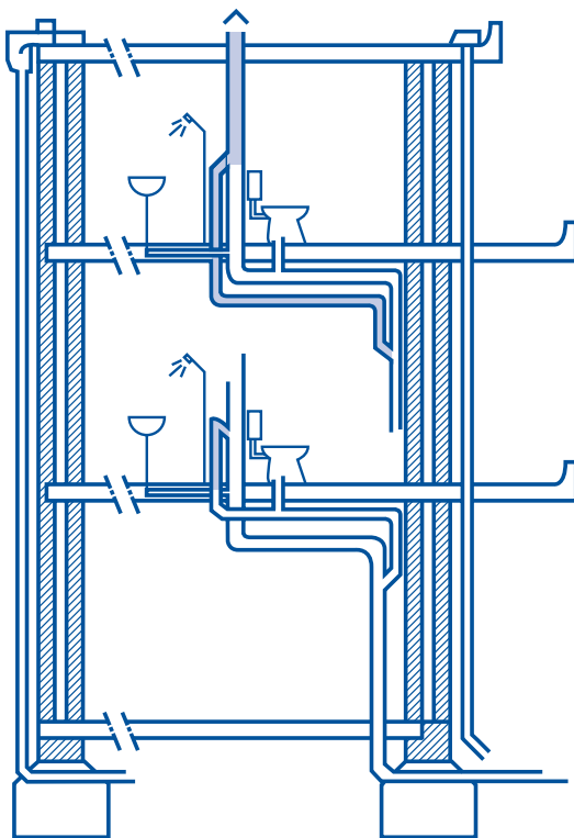
Afb. 4.5 Voorbeelden van een vereveningsleiding.
