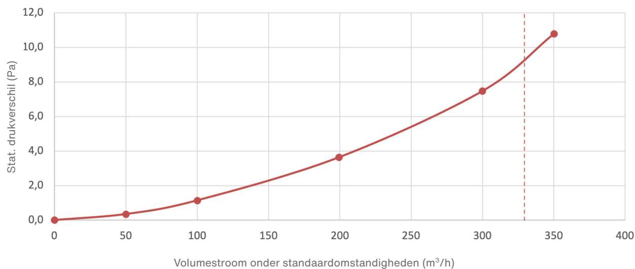
Afvoerlucht DN160
