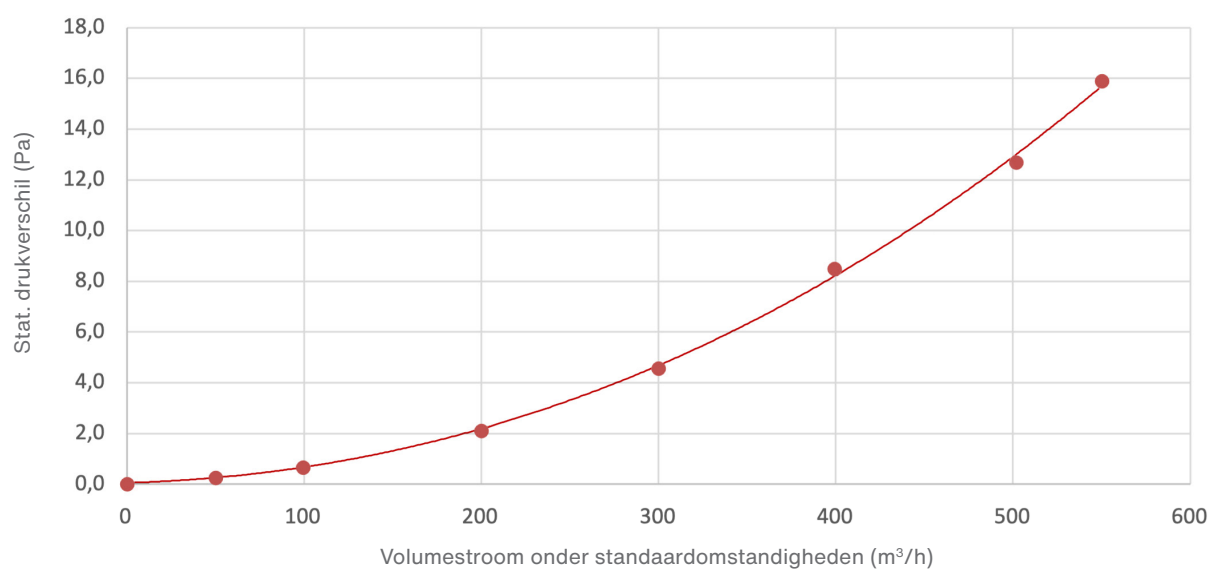
Afvoerlucht DN200
