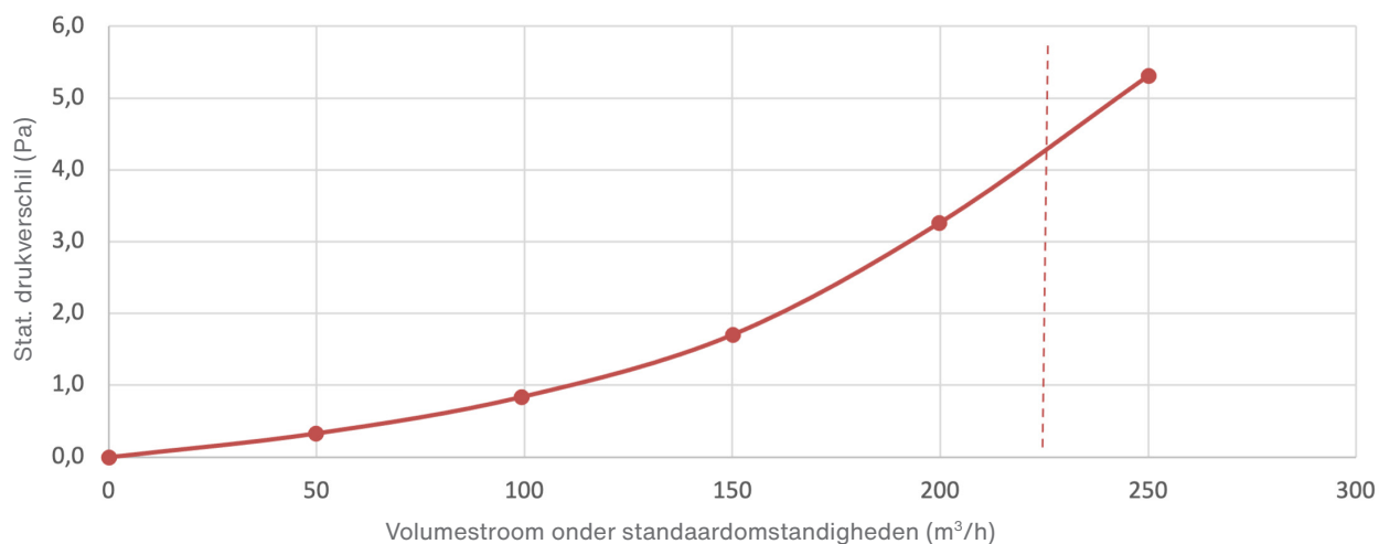
Afvoerlucht DN125
